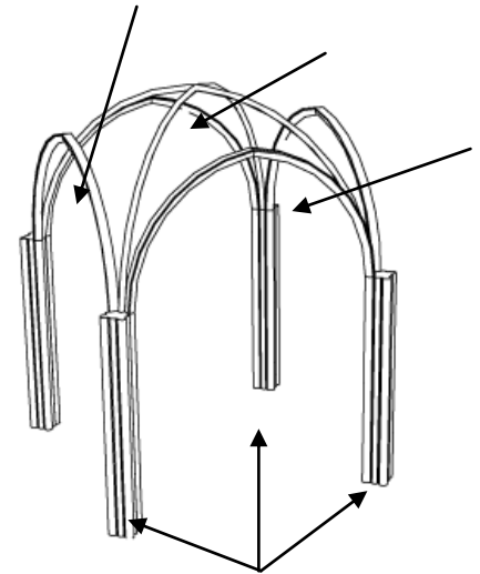
Bóveda de crucería simple (cuatripartita: 4 plementos)
