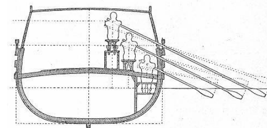
Sección de una trirreme griega
